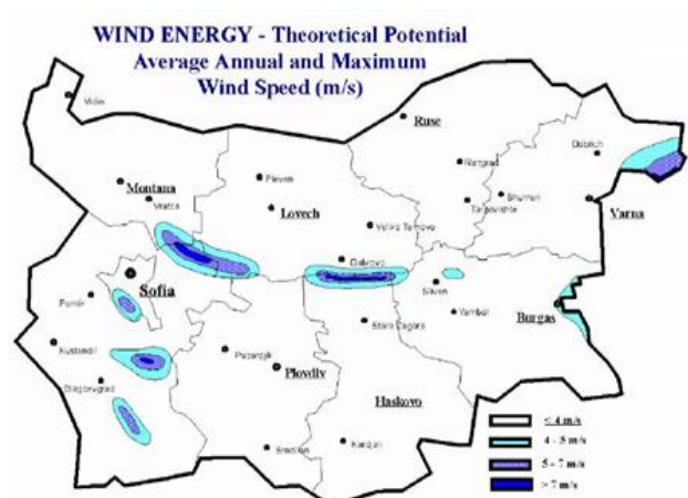
КАРТА 5. КАРТОСХЕМА НА ВЕТРОВИЯ ПОТЕНЦИАЛ В БЪЛГАРИЯ
